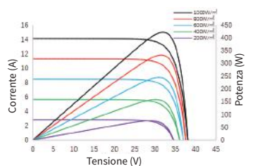
Curva corrente/potenza-tensione SS8-54HDB-420N
