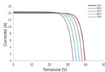
Curva corrente-tensione SS8-54HDB-420N
