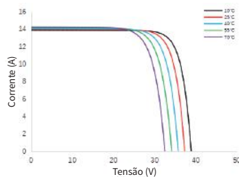
Curva de corrente e tensão SS8-54HSB-410M
