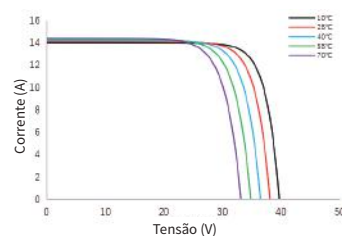
Curva de corrente e tensão SS8-54HD-420N
