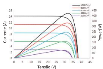
Curva de corrente/potência-tensão SS8-54HD-420N
