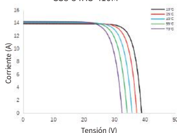
Curva de corriente- tensión SS8-54HS-410M
