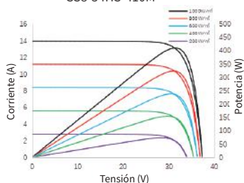
Curva de corriente/potencia-tensión SS8-54HS-410M
