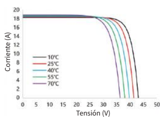
Curva de corriente- tensión SS9-60HS-600M
