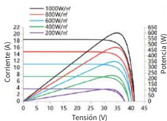
Curva de corriente/potencia-tensión SS9-60HS-600M
