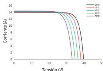
Curva de corriente- tensión SS8-54HDB-420N
