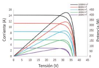
Curva de corriente/potencia-tensión SS8-54HDT-420N
