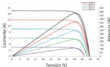
Curva de corriente/potencia-tensión SSA-66HD-610N
