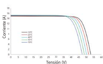
Curva de corriente- tensión SSA-66HD-610N
